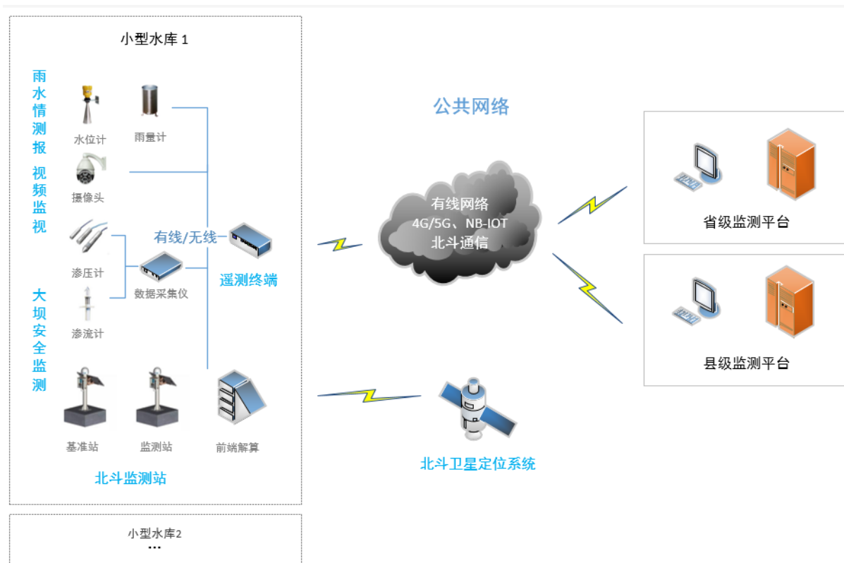
图 2.1 水库雨水情测报和大坝安全监测系统总体架构图
