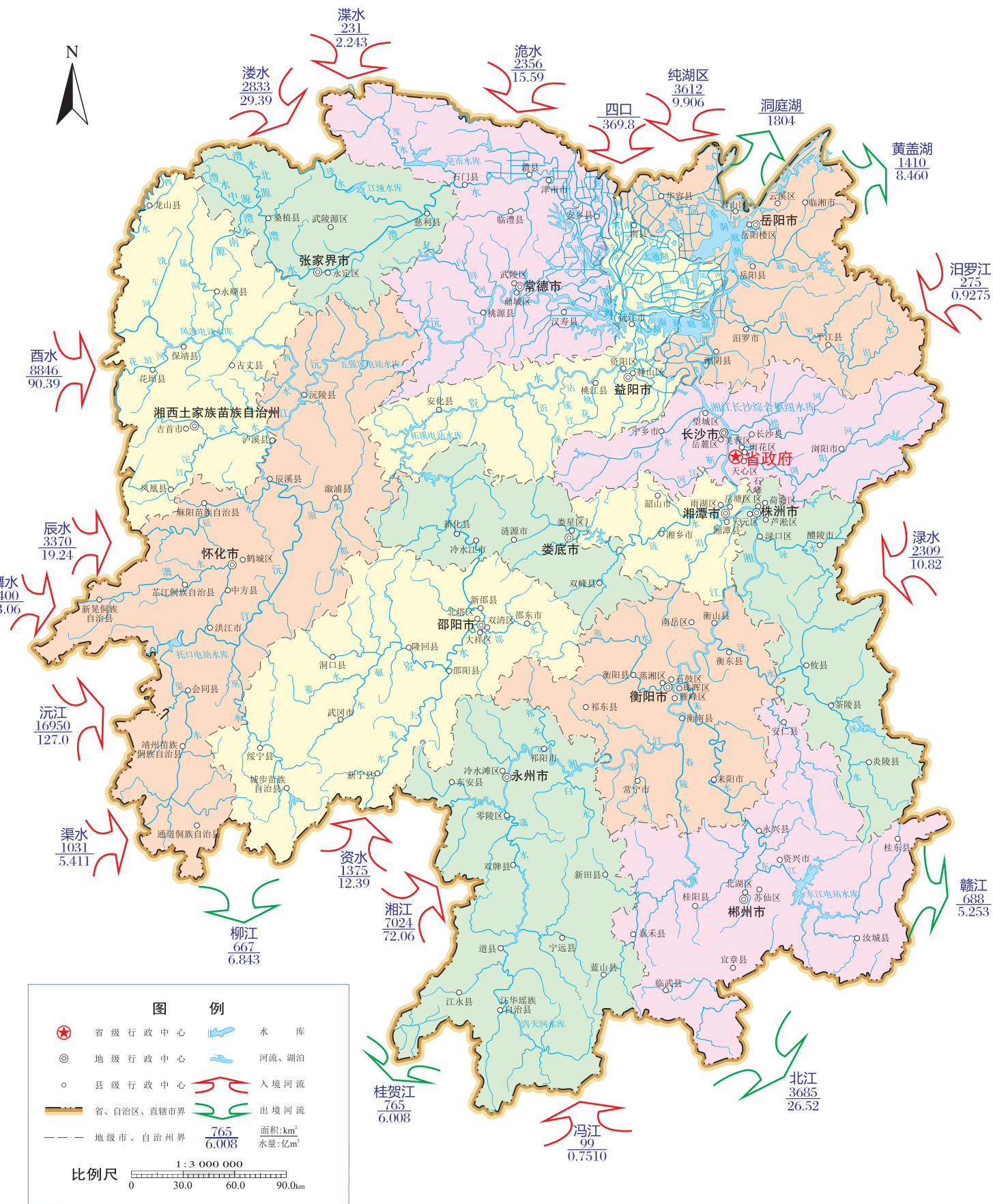
图 11 2025 年全省入出境水量示意图
